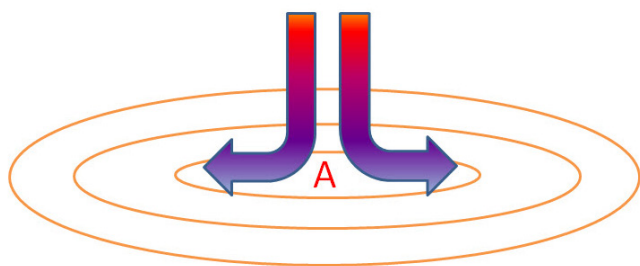
Figura 36: Diagrama de moviments de vent en anticicló. Font: BCNecologia.
