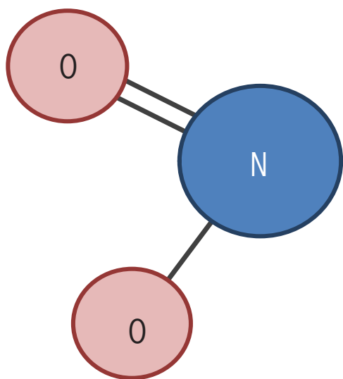
Figura 1: Molècula de diòxid de nitrogen ( \text{NO}_2 ).
