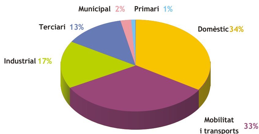
Emissions de GEH per sectors, 2006
