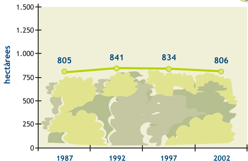
Evolució de la superfície forestal de Sabadell
